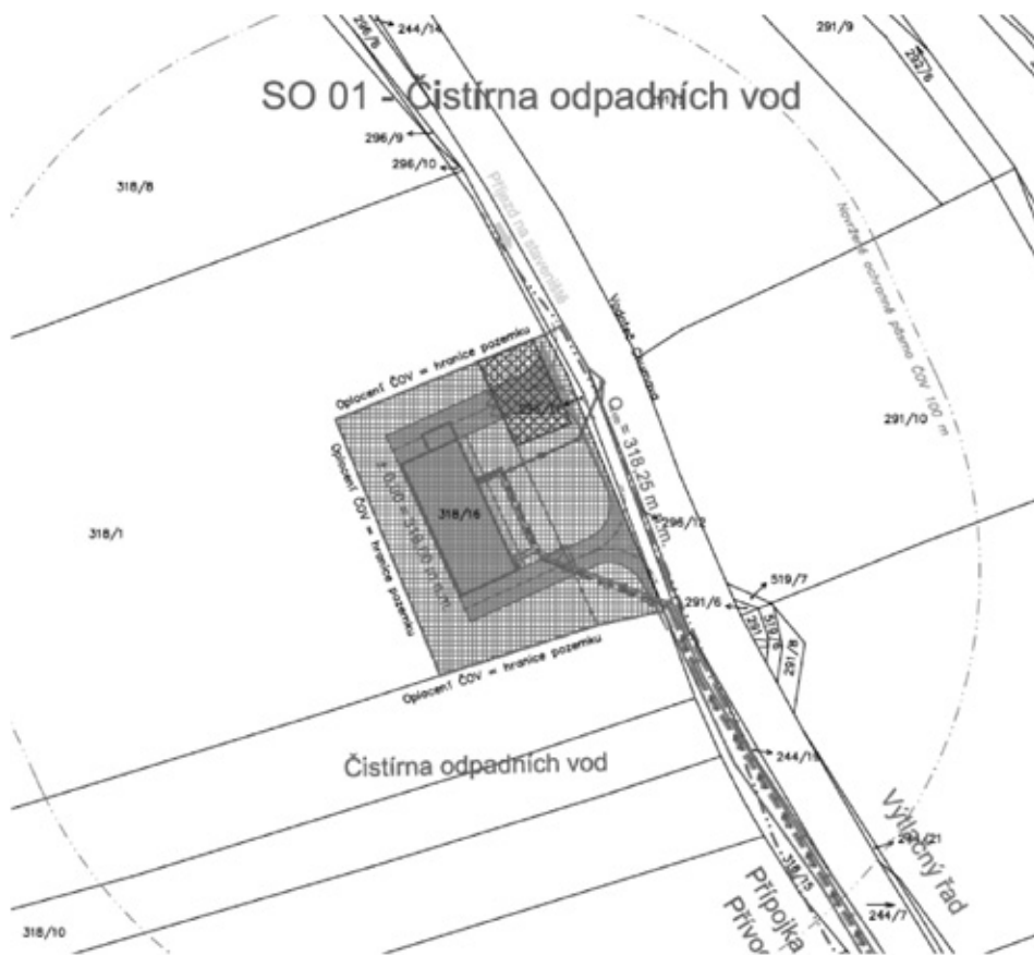
Obrázek 1: výřez z Celkového situačního výkresu stavby
